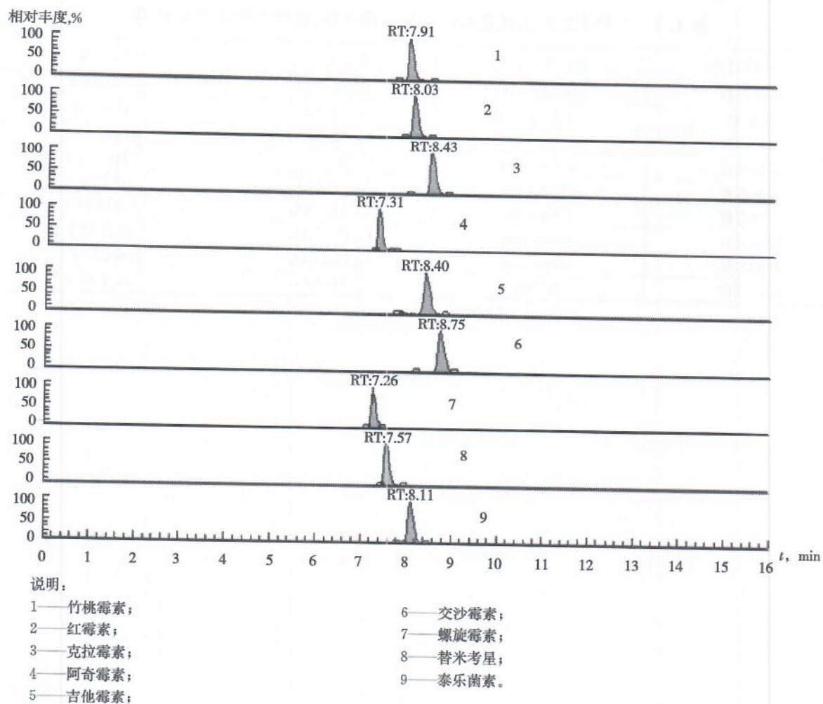
图 B.1 大环内酯类药物混合标准溶液(1 ng/mL)的特征离子质量色谱图
